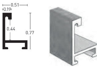
Profil 273 Natura | Profile 273 Natura
