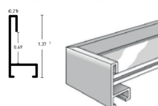
Profil 34 Natura | Profile 34 Natura
